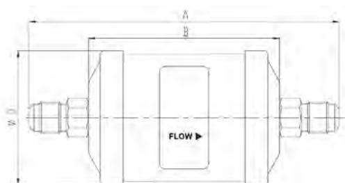
Conexão Rosca
