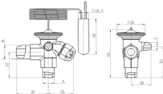
Corpo válvula - Tipo de conexão: rosca / rosca / rosca
