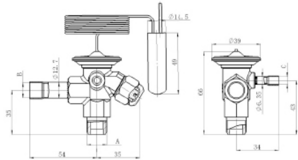
Corpo válvula - Tipo de conexão: rosca / solda / solda
